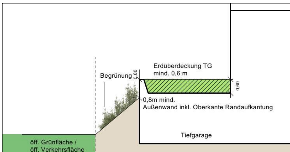
Schemaschnitt (unverbindlich) „Anböschung“
