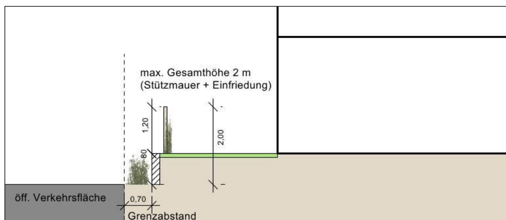
Schemaschnitt – Abstand und Gesamthöhe von Einfriedungen (inkl. Stützmauer)
