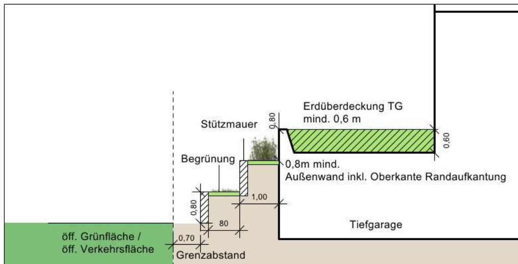
Schemaschnitt (unverbindlich) „Abtrepung“ von Stützmauern
