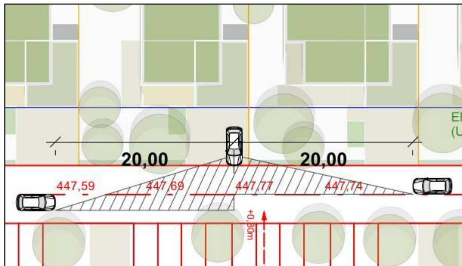
Schema Sichtdreieck
